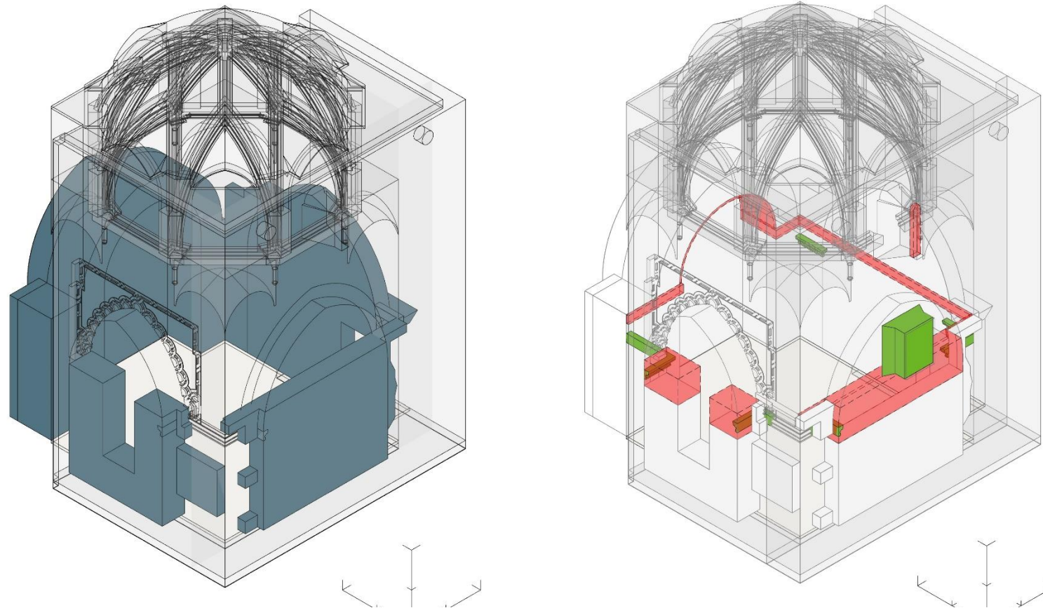
Esquema de trabajo: discretización del modelo y asignación de propiedades.
